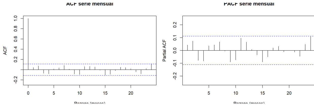
Figura 6. ACF y PACF de la serie mensual de conteos del catálogo.
